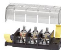
BLUE SEAS Bloque de fusibles MRBF con fuente independiente, 240A por circuito, 3 pernos Ref: 5194-BSS Ver más >
