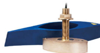
RAYMARINE Transductor pasacascos bronce B275LH, 1000W, para sonda Chirp Ref: A80322 Ver más >
