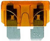
BEP MARINE Fusible de 25 Amp JAP tipo cuchilla Ref: J25A Ver más >
