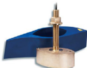
RAYMARINE B260, Transductor prof/temp pasacascos bronce, 1KW 50/200 kHz con barquilla, para CP370 Ref: E66079 Ver más >
